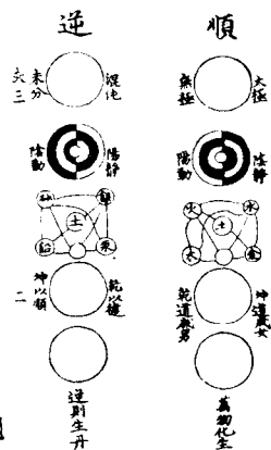
圖象體氣元圖逆順極太
