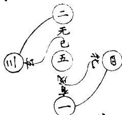
圖一五三丹金
