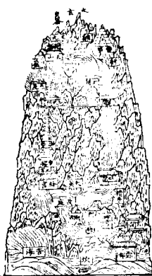
圖象體氣元圖逆順極太
