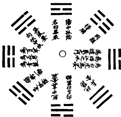
圖之卦八丹金
