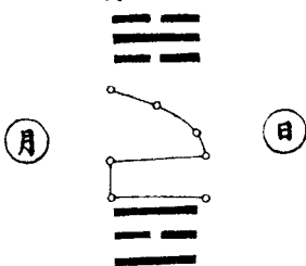
圖之象四丹金
